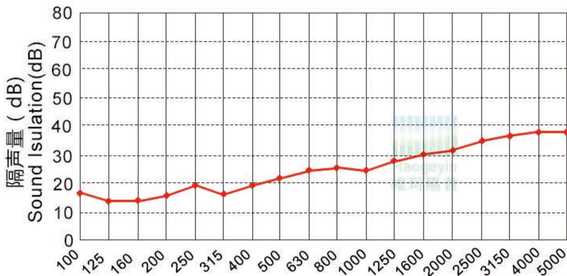
阻尼隔音毡隔音数据测试图
